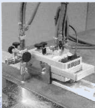
IMP za automatsko ravno rezanje pod nepravilnim kutevima
