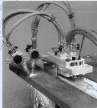
IMP sa jednostrano postavljenim plamenicima za rezanje bridova
