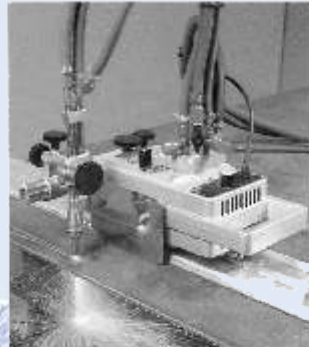
IMP za automatsko ravno rezanje pod nepravilnim kutevima
